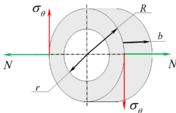
Рисунок 5. Схема отрезка от шлифовального барабана.
