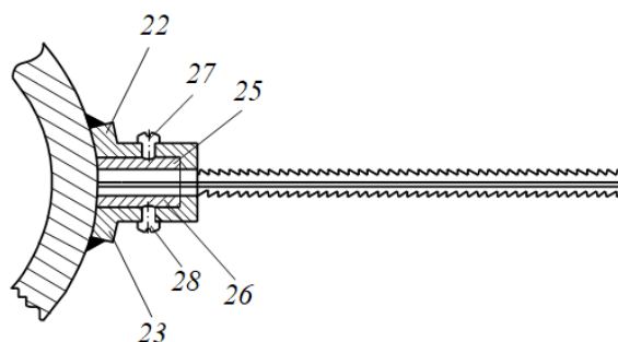
Рисунок 3. Крепление шлифовальной бумаги к барабану. Attachment of abrasive paper to the grinding drum.
