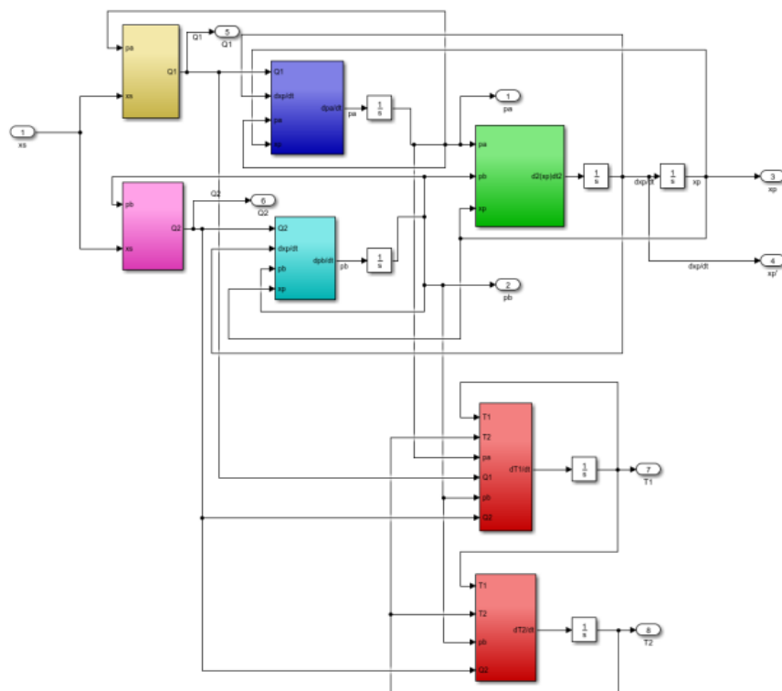
Рисунок 4. Схема математической модели гидросистемы с учётом изменения температуры.
