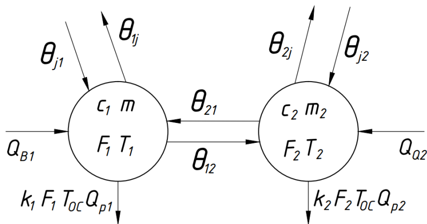
Рисунок 2. Схема внутреннего теплообмена в гидросистеме.
