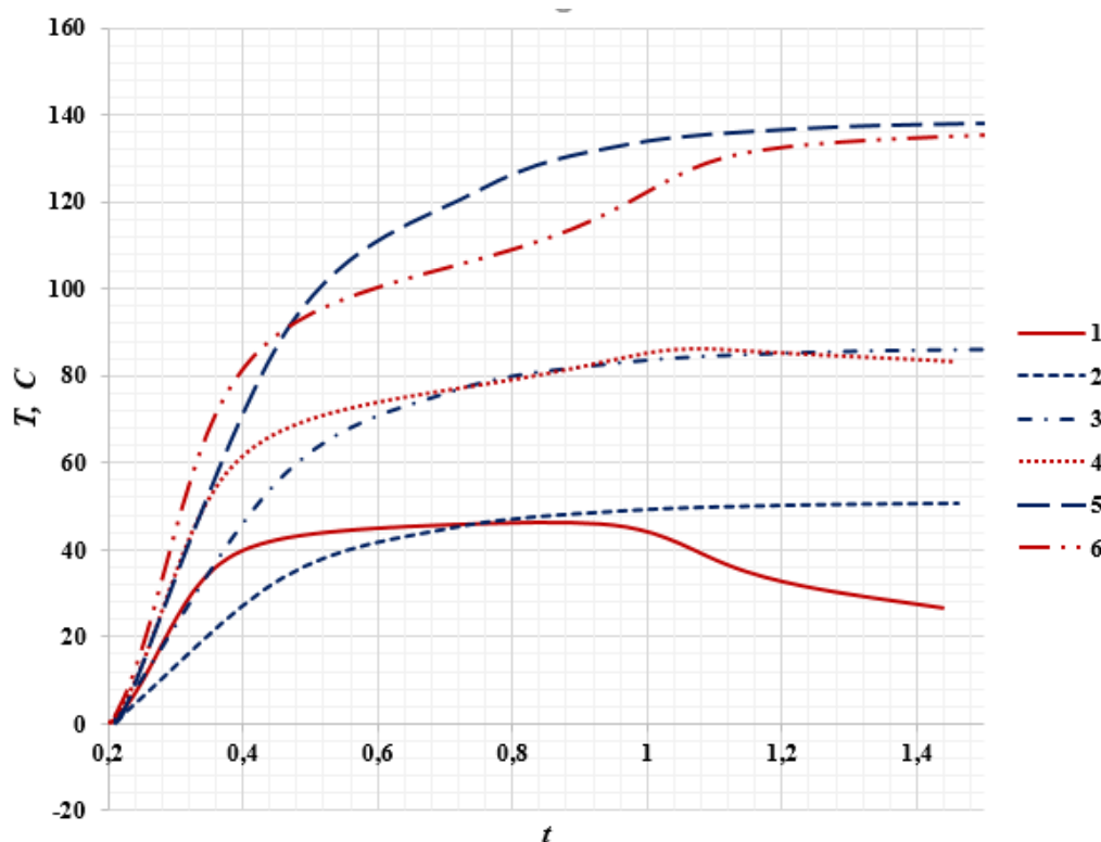
Рисунок 7. Сравнение изменений температуры в гидравлической системе, соответствующей участку I.
