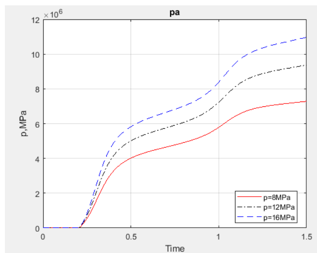
Рисунок 5. Временная реализация давлений p_A в поршневой части гидроцилиндра.
