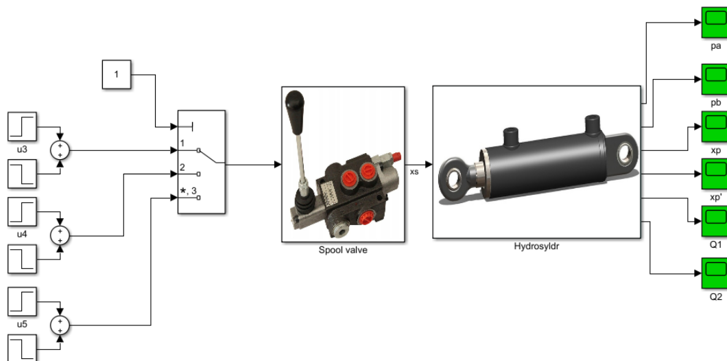
Рисунок 3. Общий вид Simulink-модели гидросистемы.
