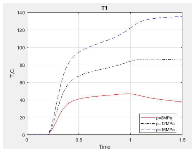
Рисунок 6. Временная реализация температуры T_1 , соответствующая участку I гидросистемы.
