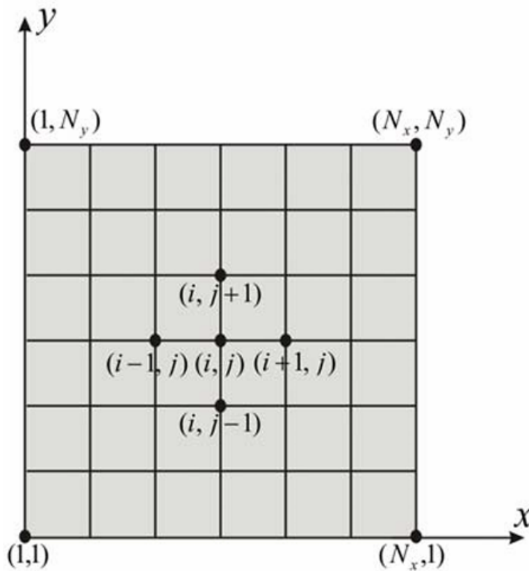
Рисунок 2. Разностная сетка области решения.
