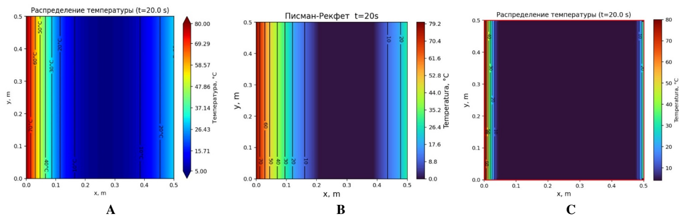
Рисунок 3. Изотермы ( ^{\circ}\text{C} ) в пластине при t = 20 с: А — FreeFEM++; В — метод Писмена–Рэчфорда; С — полуявный метод.
