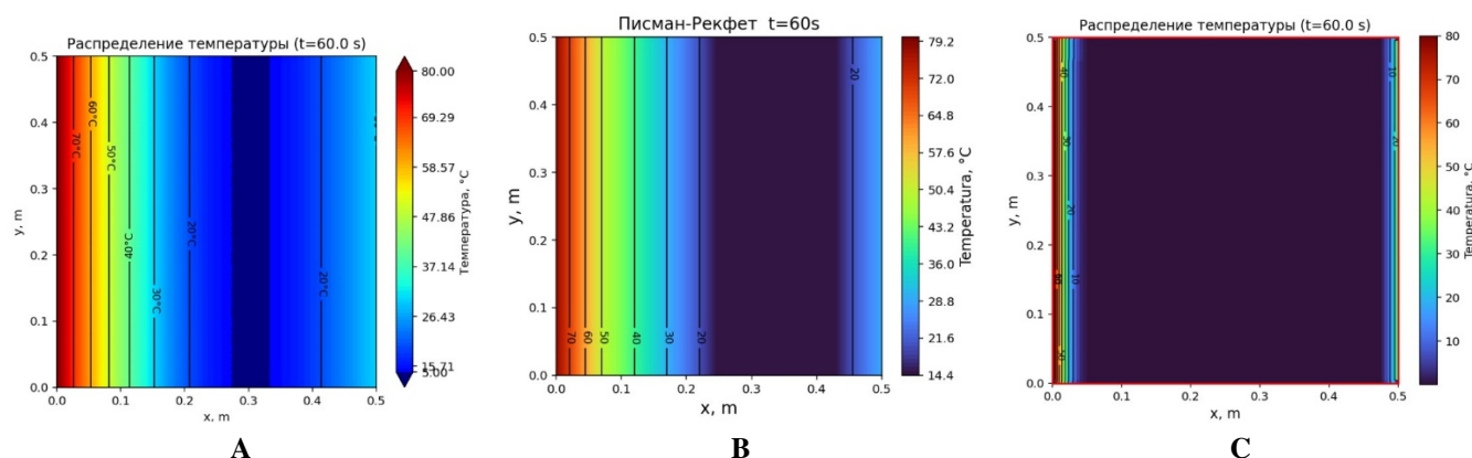
Рисунок 5. Изотермы ( ^{\circ}\text{C} ) в пластине при t = 60\text{ c} : А — FreeFEM++; В — метод Писмена–Рэчфорда; С — полуявный метод.
