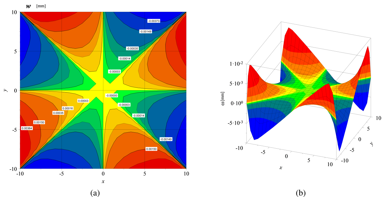
Рисунок 2. Поле деформации квадратного сечения при совместном кручении и осевом нагружении M-N : (a) контурное; (b) пространственное представление. Warping field of a square cross-section under combined axial and torsional loading: (a) contours; (b) 3D representation.
