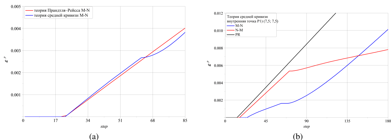
Рисунок 4. Пластическая деформация \varepsilon^P в точке P_1 : (a) модель Прандтля–Рейсса и теория средней кривизны при M \rightarrow N ; (b) теория средней кривизны для MN , NM и пропорционального нагружения (PR). Абсцисса — расчётный шаг.
