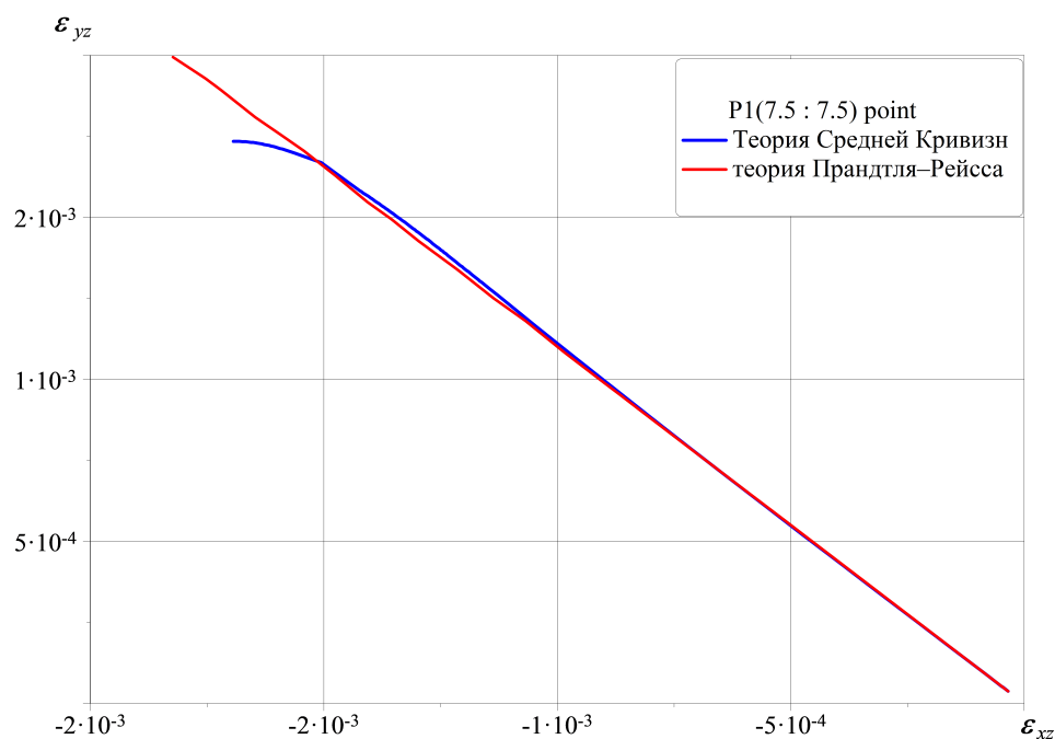
Рисунок 3. Траектории сдвиговых деформаций в точке P_1 : теория средних кривизн и модель Прандтля–Рейсса согласно обозначениям исходного графика. Shear strain paths at point P_1 : average-curvature theory and the Prandtl–Reuss model (as labelled in the original graph).
