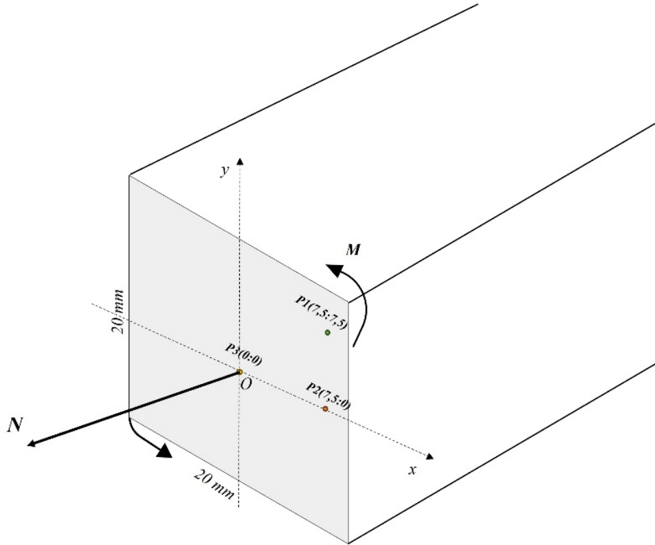
Рисунок 1. Квадратный стержень, силовые факторы N , M и контрольные точки P_1(7.5, 7.5) , P_2(7.5, 0) , P_3(0, 0) ; координаты в мм.
