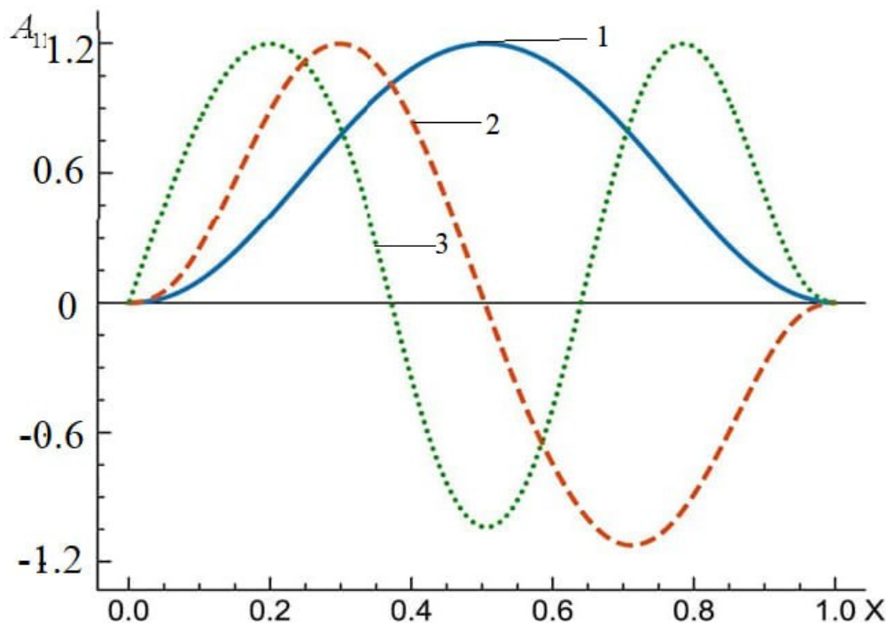
Рисунок 2. Смещения для первых трех мод колебаний: 1 — первая мода, 2 — вторая мода, 3 — третья мода Displacements for the first three vibration modes: 1 — first mode, 2 — second mode, 3 — third mode
