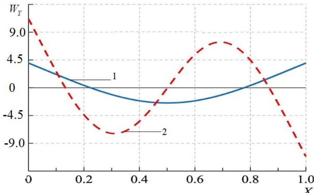
Рисунок 3. Деформация изгиба для первых двух мод колебаний: 1 — первая мода, 2 — вторая мода, 3 — третья мода Bending deformation for the first two vibration modes: 1 — first mode, 2 — second mode, 3 — third mode
