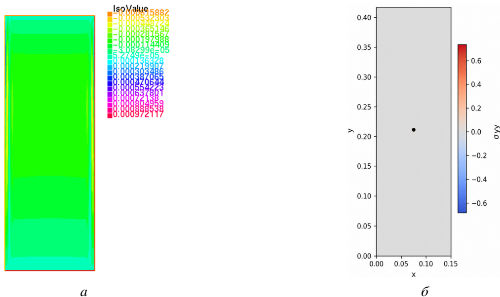
Рисунок 3. Распределение нормального напряжения \sigma_{22} в прямоугольной области в момент времени t = 0,004 с Distribution of normal stress \sigma_{22} in the rectangular domain at t = 0.004 s
