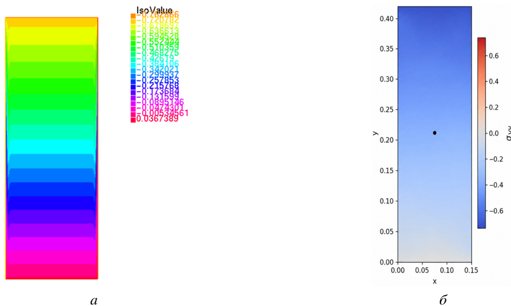
Рисунок 1. Распределение нормального напряжения \sigma_{22} в прямоугольной области в момент времени t = 0,0001 с Distribution of normal stress \sigma_{22} in the rectangular domain at t = 0.0001 s
