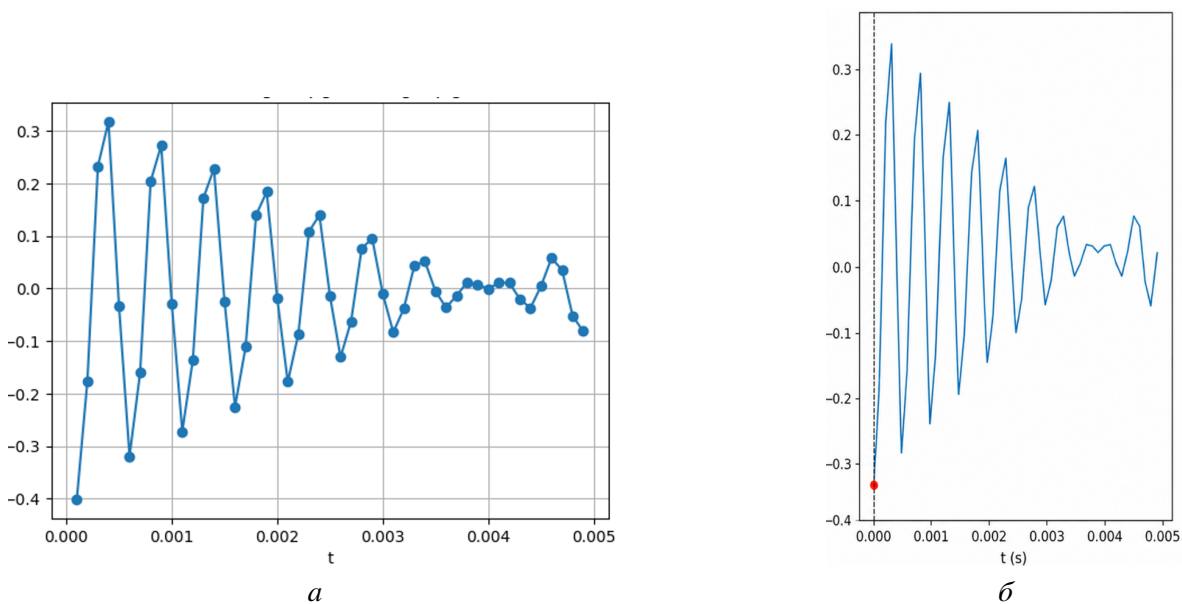
Рисунок 4. Изменение нормального напряжения \sigma_{22} во времени в центральной точке прямоугольной области Time history of normal stress \sigma_{22} at the centre of the rectangular domain
