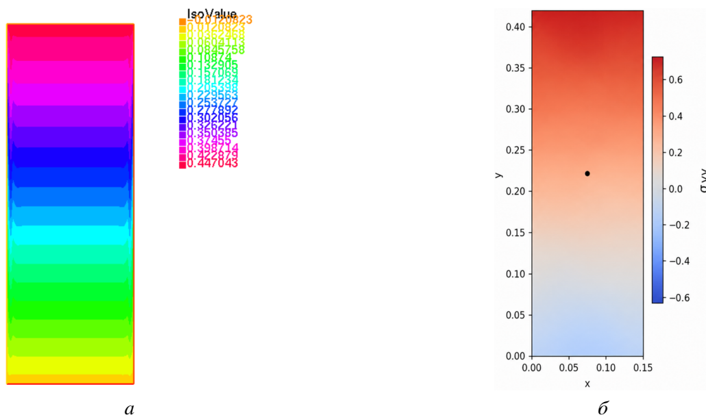
Рисунок 2. Распределение нормального напряжения \sigma_{22} в прямоугольной области в момент времени t = 0,0003 с Distribution of normal stress \sigma_{22} in the rectangular domain at t = 0.0003 s
